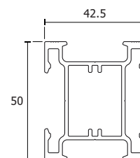
Viga de Aluminio Medidas: 42.5x50 mm Largo máx. 5.80 m
