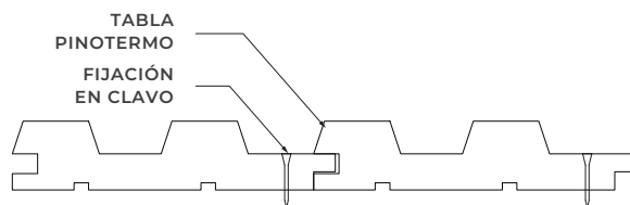
Sección transversal Detalle unión entre tablas.
