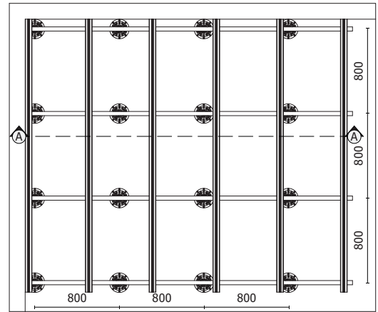
PLANTA N +0.00
