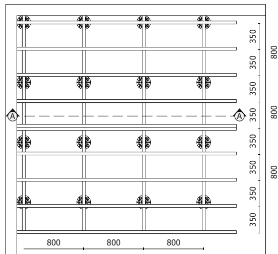
PLANTA N +0.00
