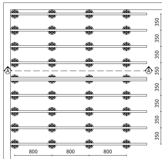
PLANTA N +0.00
